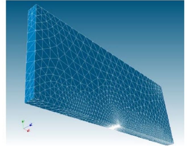
Figura 11. Malla típica de elementos finitos para modelo 3D.
